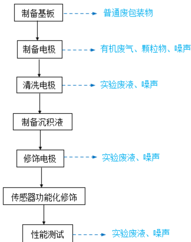
图 2-2 项目工艺流程及产污环节示意图
